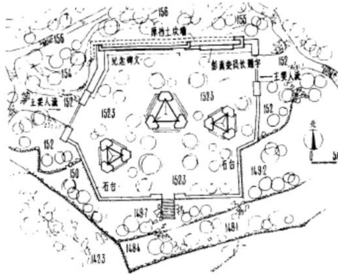
苗冠峰《一二·九运动纪念亭》中所附的纪念亭平面设计图
